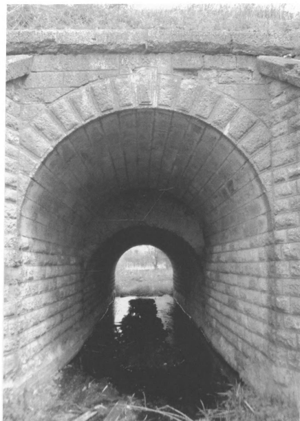
Водопропускная труба Балашовской ветки ЮВЖД вблизи станции Чакино (район д. Бабанино).
